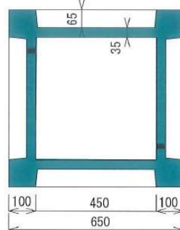
B-B断面
