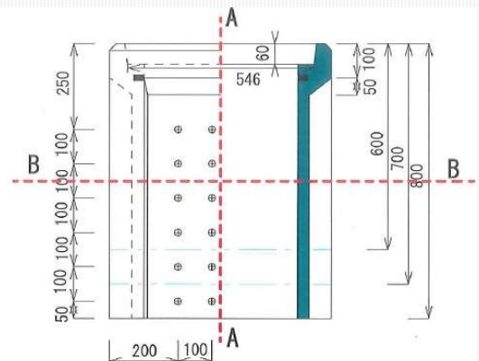
A-A断面
