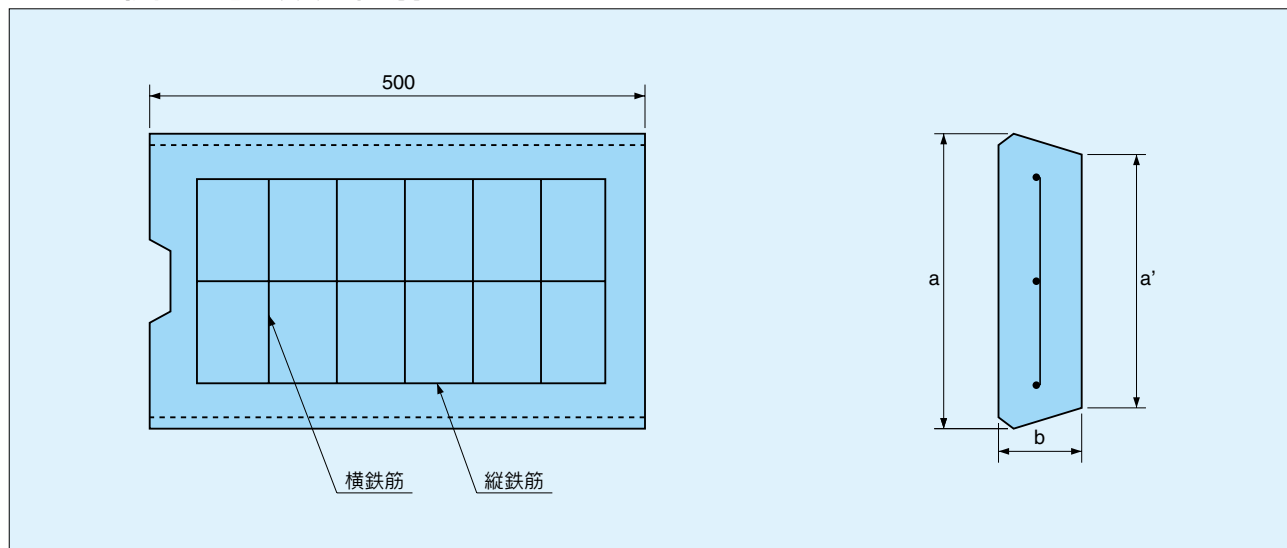
ふたの形状、寸法及び配筋 (単位: mm)
