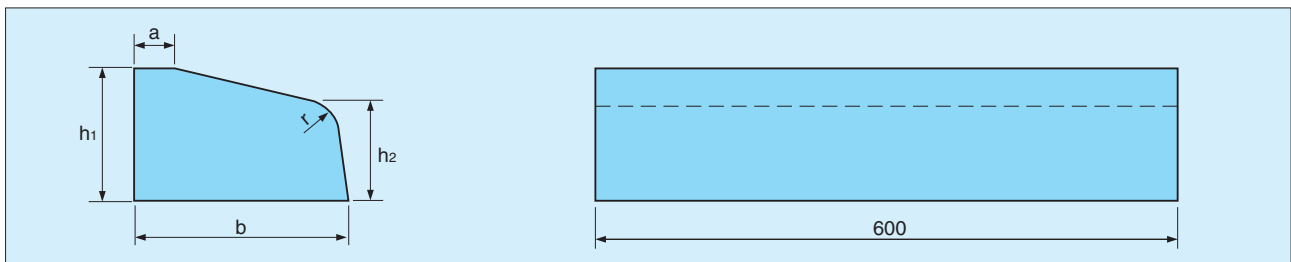
寸法・配筋・質量表
