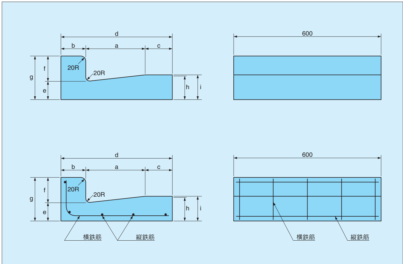
形状、寸法及び配筋 (単位：mm)
